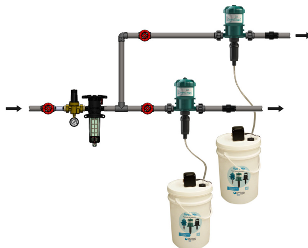
Instalação Dupla Fixa em Linha
